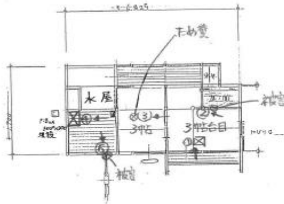
物外軒平面図 1/100
